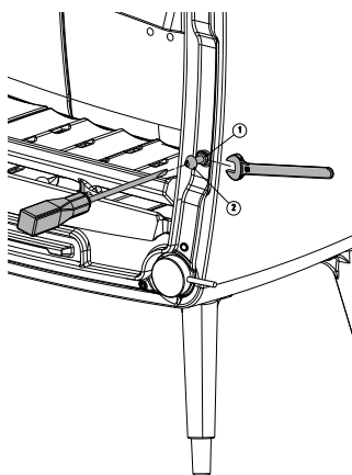
Fig. 17 Justering av dørlukker. Denne justeringen kan være nødvendig etter skifte av dørpakning eller etter en tids bruk. Blir døren hard å lukke, løsnes kontramutteren (1) og skruen (2) dreies mot venstre. Når riktig posisjon er funnet, strammes kontramutter. Er dørlukker slakk, dreies skruen i motsatt retning.
