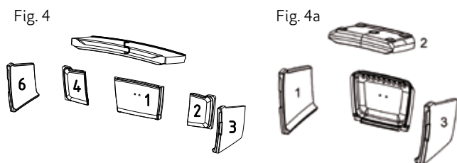
Fig. 4 Demontering/montering av steinsett Vintage 50 og 35 Ved demontering start med høyeste tall og motsatt ved montering. Når røykrør skal feies kan røykleder/hvelvplate (5) fjernes. For å kunne fjerne denne må stein (6) fjernes først og deretter røykleder (5). Sett steinene inn i motsatt rekkefølge.
